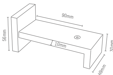
SOPORTE FRENTES STANDARD ELITE CROMO
