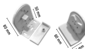
JUEGO SOPORTE ESTANDAR MÉRIDA PLUS (SET INDIVISIBLE)
