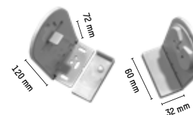
JUEGO SOPORTE LARGO 72 MM (SET INDIVISIBLE)
