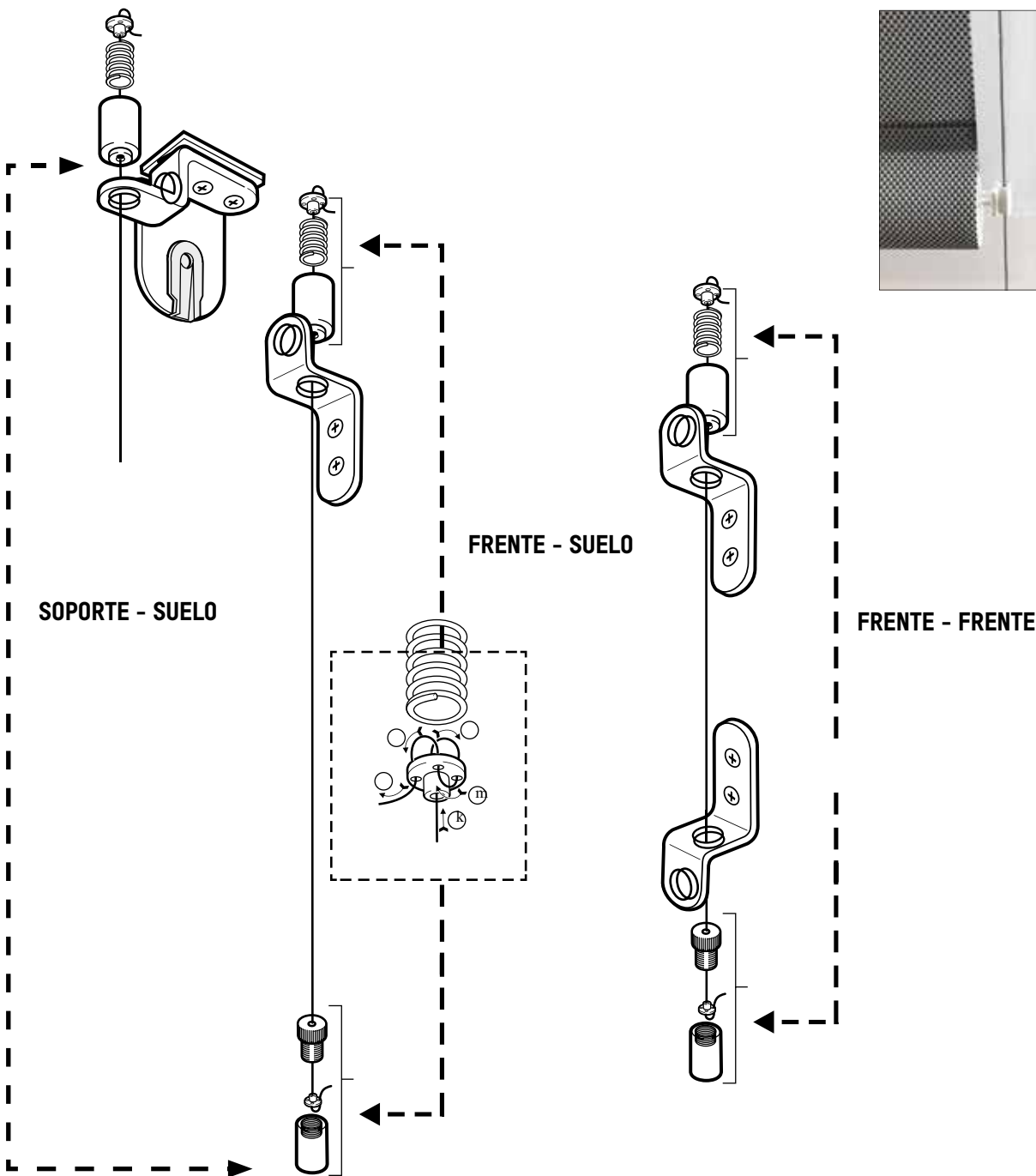
GUIADO CABLE XXL 2mm FRENTE/SUELO SOPORTE/SUELO
