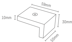
SOPORTE TECHO ELITE CROMO
