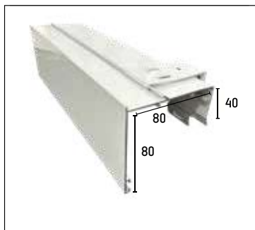
MEDIDAS PERFIL BASIC BOX
